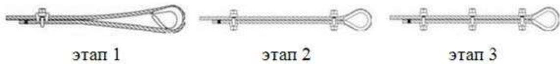
Рисунок 9 - Крепление стального троса
